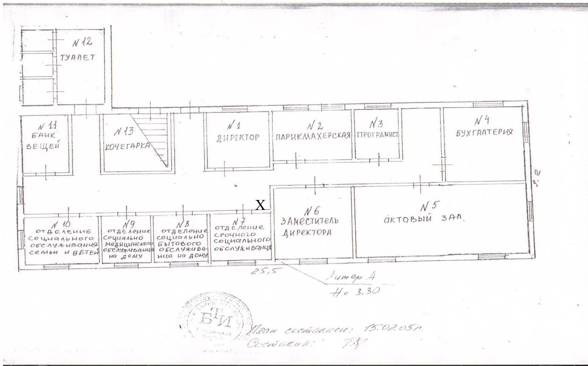
План-схема здания.
